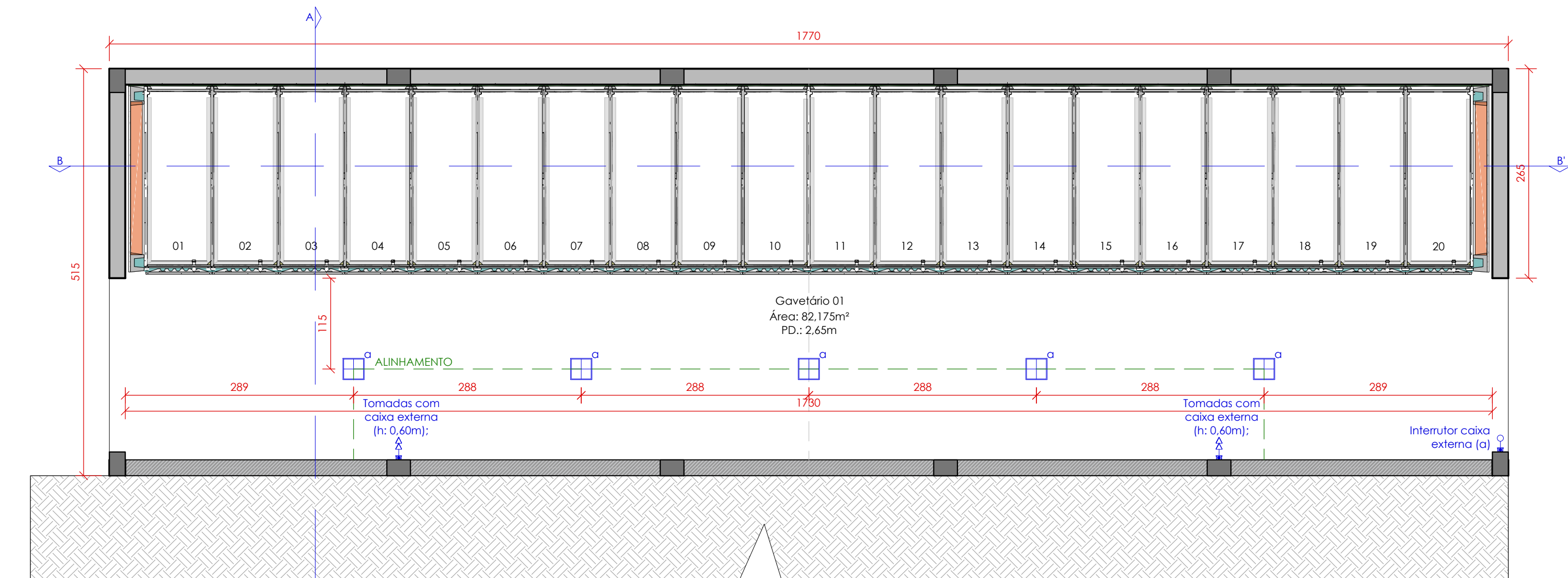
Planta Baixa - Elétrico (térreo) Esc.: 1/50
