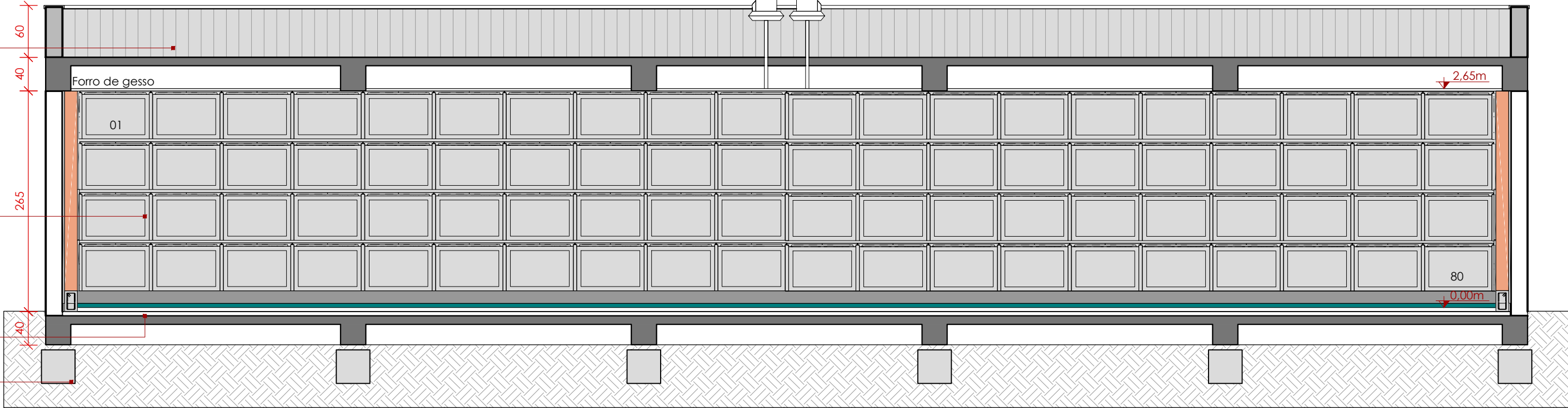
Corte BB' Esc.: 1/50
